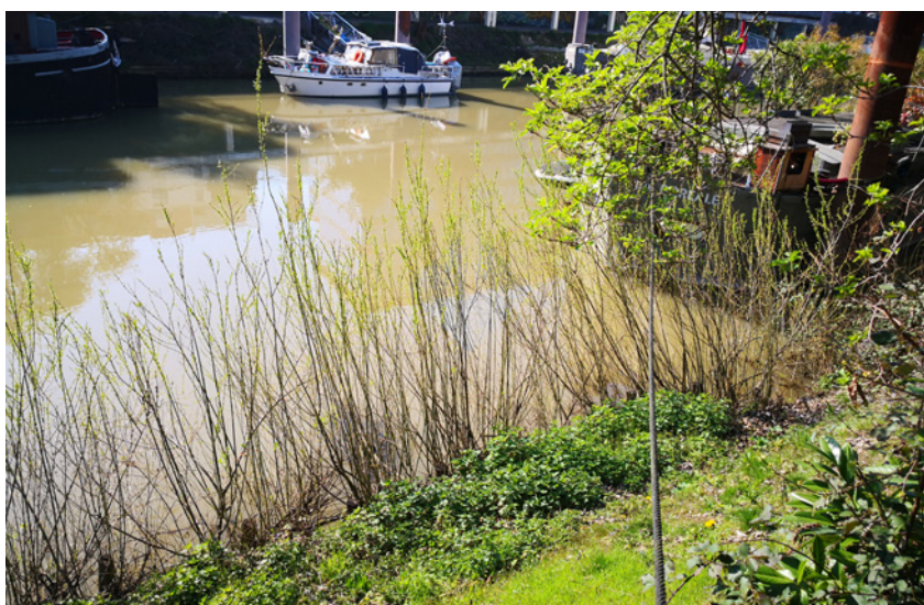
Ouvrage réalisé par l'Association Espaces en 2010 au pied du pont de Billancourt sur l'île Saint-Germain à Issy-les-Moulineaux (92). Différentes techniques issues du génie végétal ont été associées pour redynamiser la végétation et protéger durablement le talus et la berge : fascines, boutures de saules et couches de branches à rejets sous géotextile. © Association Espaces
