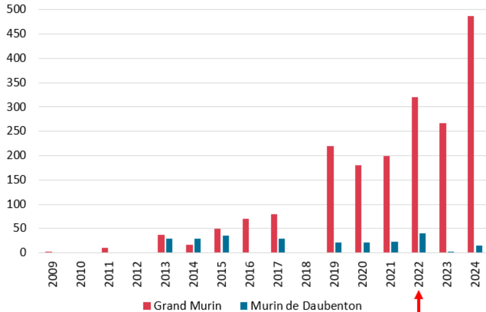
Effectifs de Grands Murins et de Murins de Daubenton en période de reproduction à Dennemont
