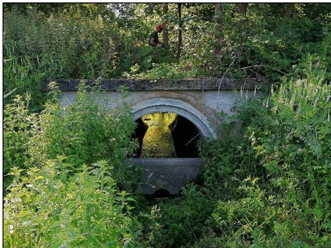
Etat initial de l'ouvrage de régulation du Bassin (vue amont)
